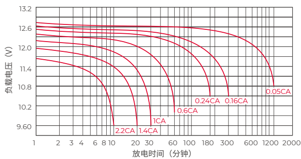
放电特性曲线
